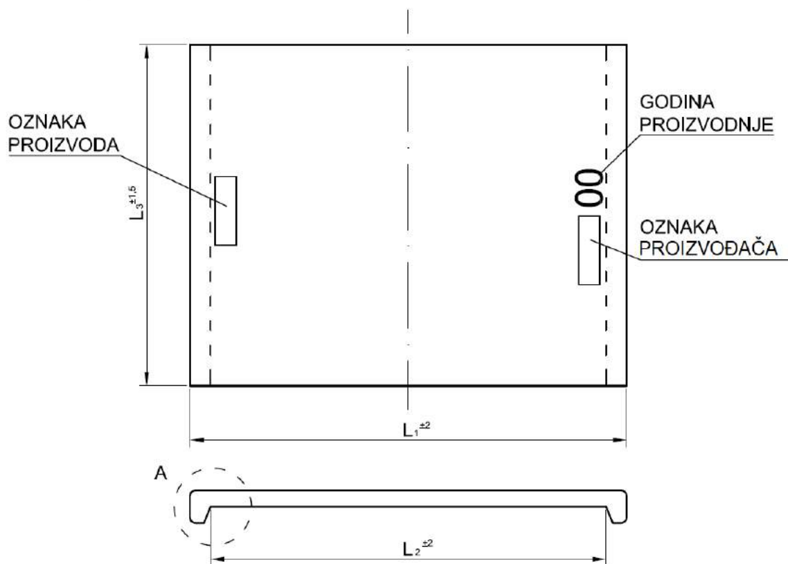
DETALJ 'A'
